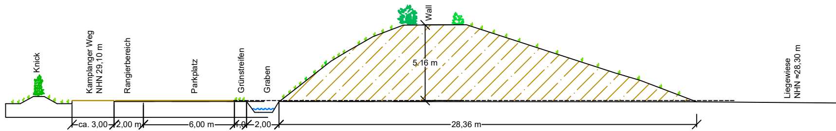
Teil A2: Schnitt A-A' M 1: 250
